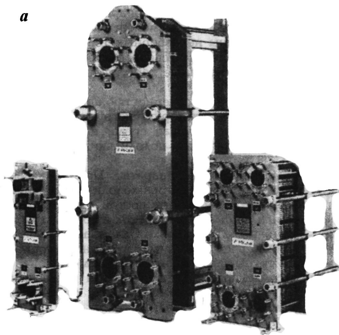
Рис. XXII-18. Пластинчатые теплообменники фирмы "Alfa Laval": а — разборные; б — паяные
